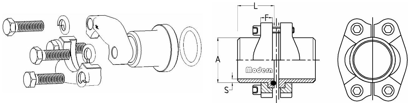
B 类-对半法兰组件-高压
