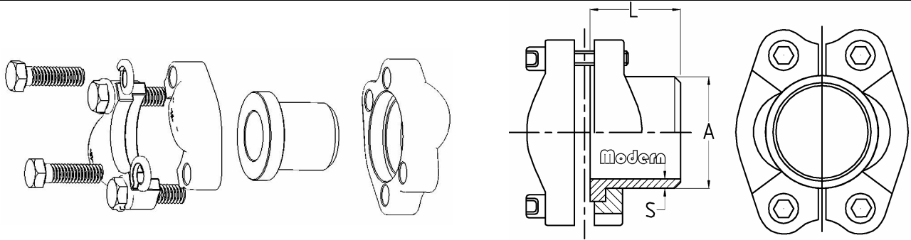
C 类-对半法兰组件-标准压力
