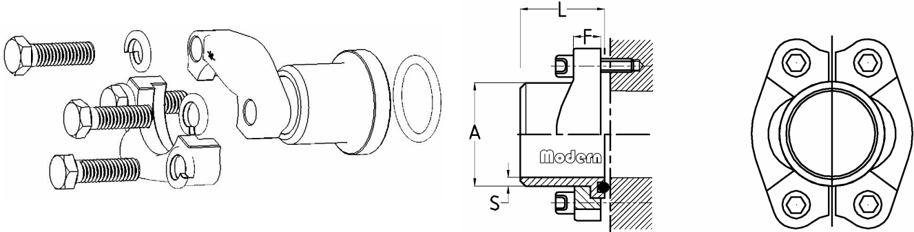
A 类-对半法兰组件-高压
