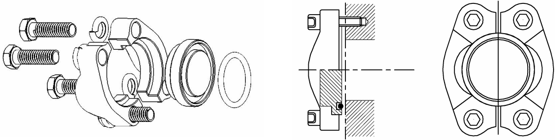
E 类-对半法兰组件-标准压力
