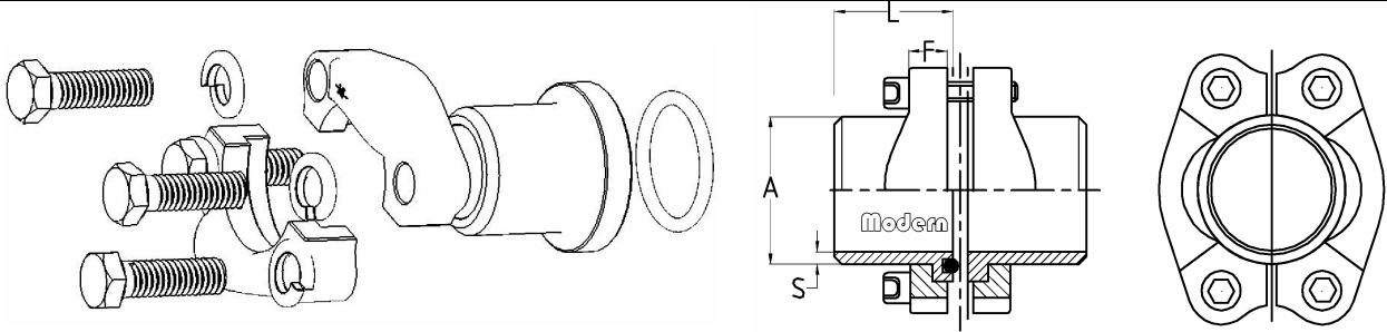
B 类- 对半法兰组件-标准压力
