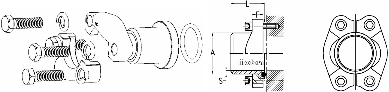
A 类-对半法兰组件-标准压力
