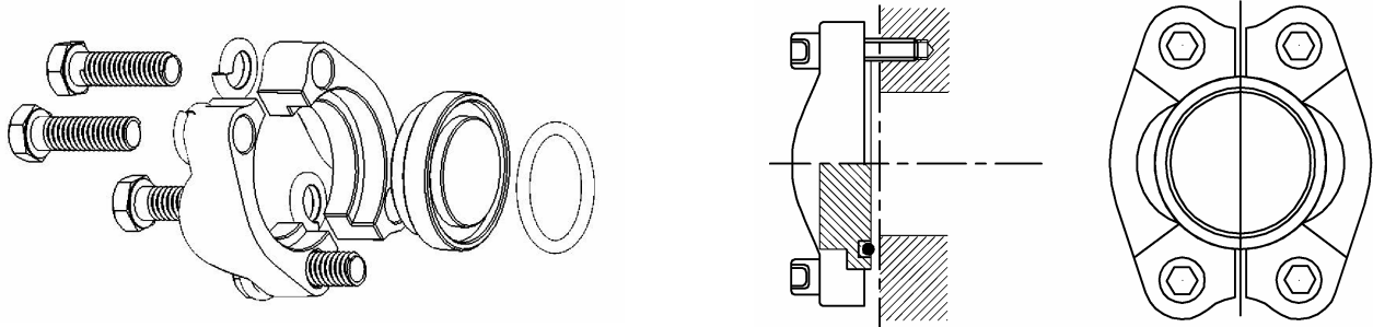
E 类-对半法兰组件-高压
