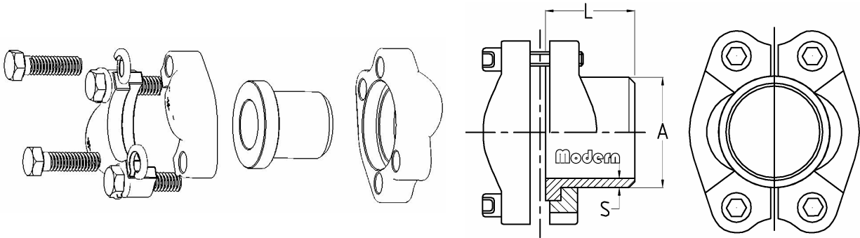
C 类-对半法兰组件-高压
