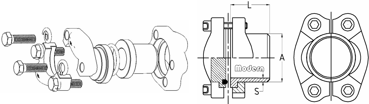
D 类-对半法兰组件-高压
