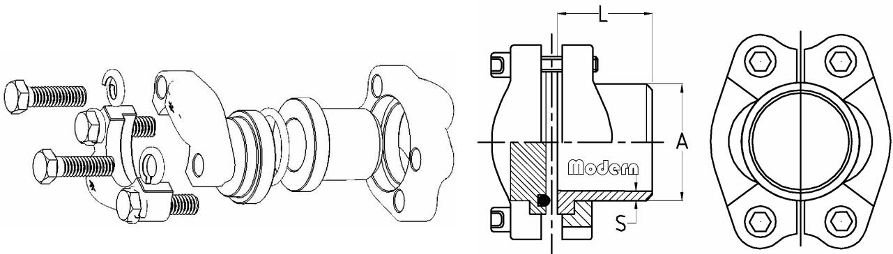
D 类-对半法兰组件-标准压力
